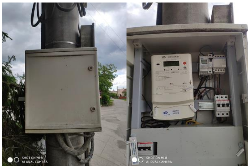
Obr. 12 Rozvádzač č. 5
